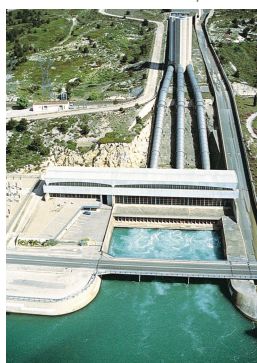
Centrale hydroélectrique de Saint-Chamas, Marseille
